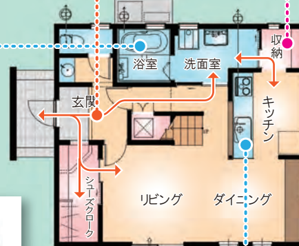
1F 平面図
